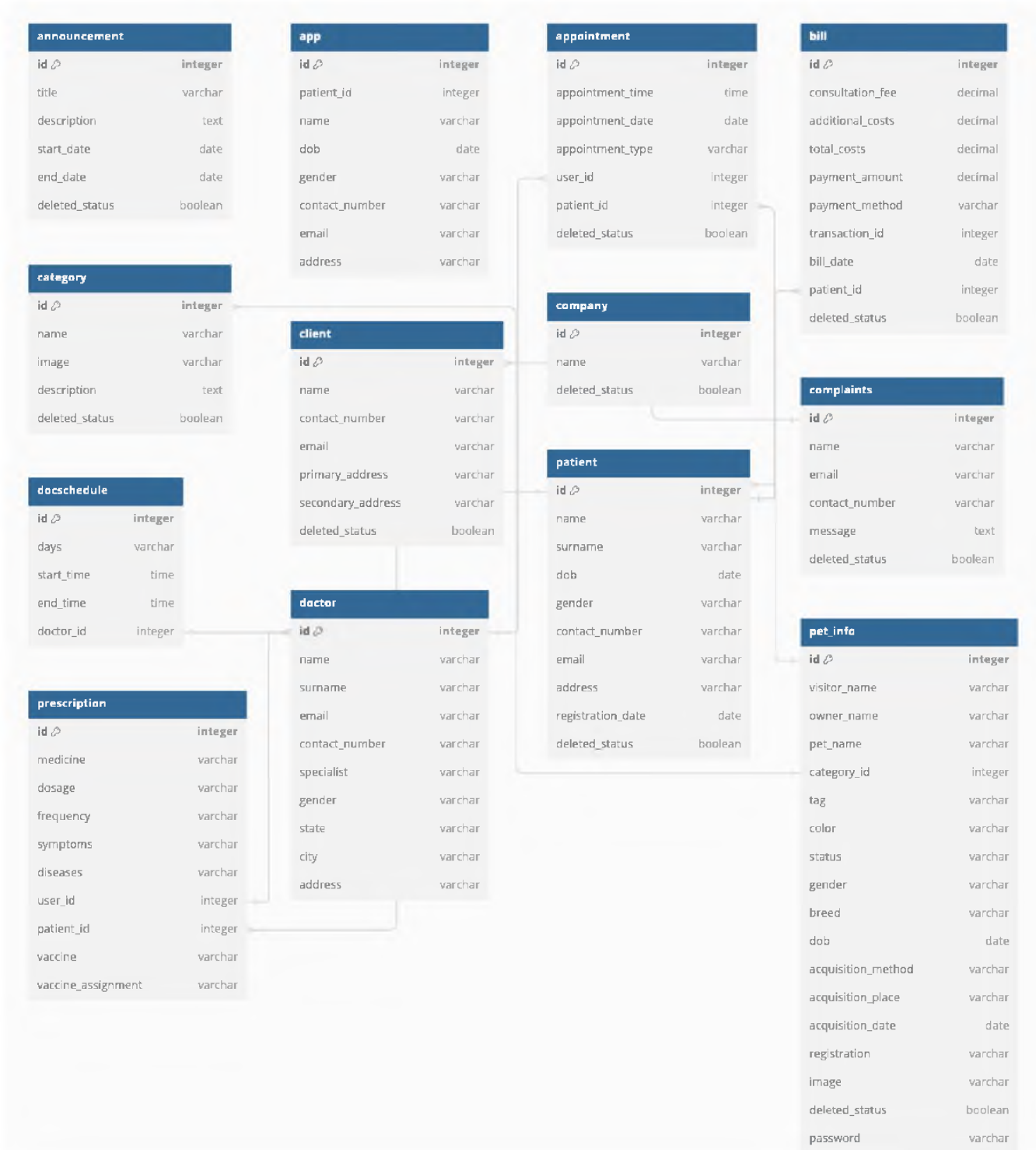
Рис.14 . Діаграма зв'язків між сутностями бази даних
