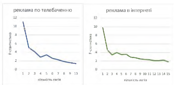
Рис. 2. Графіки значень F-статистик причинової за Гренджером залежно від кількості лагів у моделі
