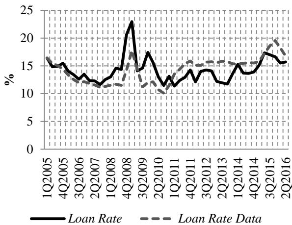
Рис. 4. Відтворення моделлю системної динаміки рівня процентних ставок за кредитами ( Loan Rate ) у порівнянні з історичними даними ( Loan Rate Data )
