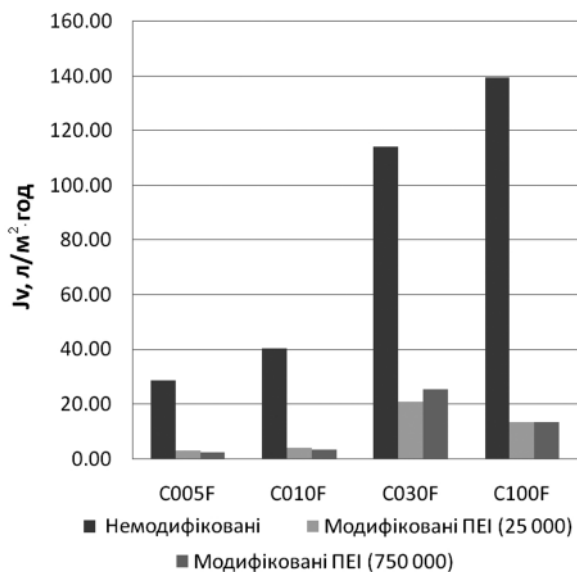
Рис. 2. Об’ємний потік води крізь мембрани, модифіковані PEI, різної молекулярної маси ( \Delta P = 0,5 мПа для мембран C100F і C030F та 2 мПа для C010F і C005F)
