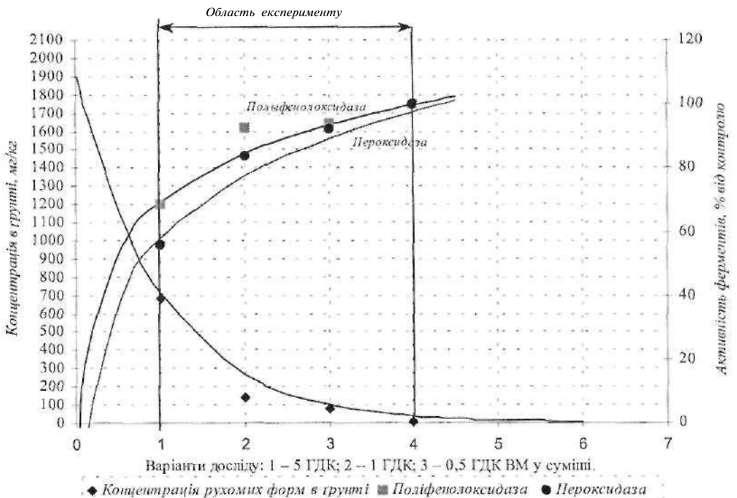
Рис. 2. Діапазон активності оксидаз в умовах мультиметалічного імпактного забруднення на чорноземі типовому малогумусному.
