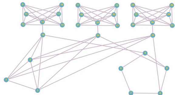
Рис. 3. Граф G_1
