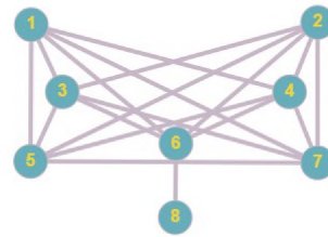
Рис. 2. Граф \tilde{H}_5
