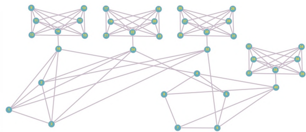
Рис. 4. Граф G_2
