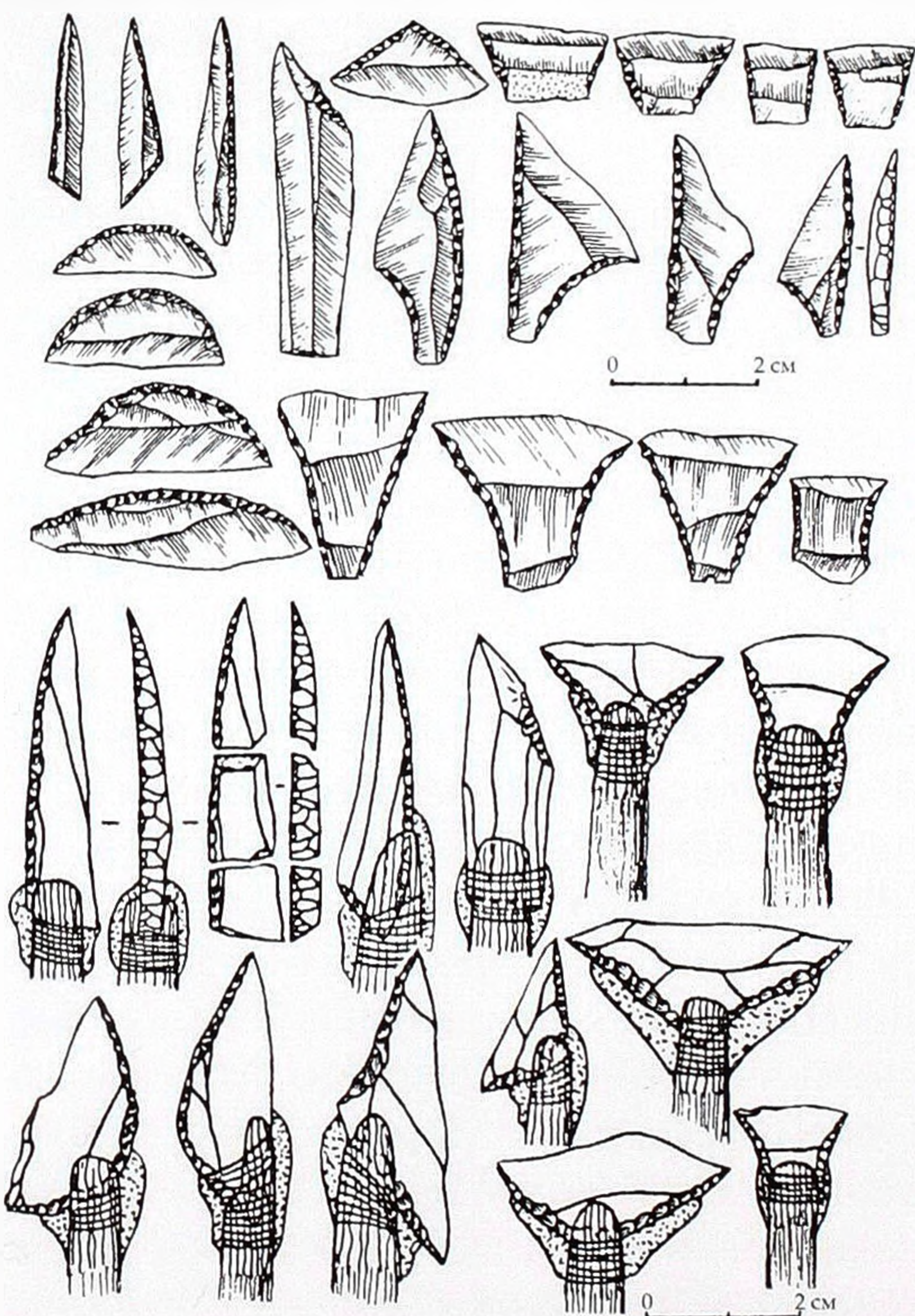
Рис. 22. Крем'яні наконечники стріл у формі геометричних мікролітів (трикутників, трапецій, сегментів) і способи їх закріплення на деревку
