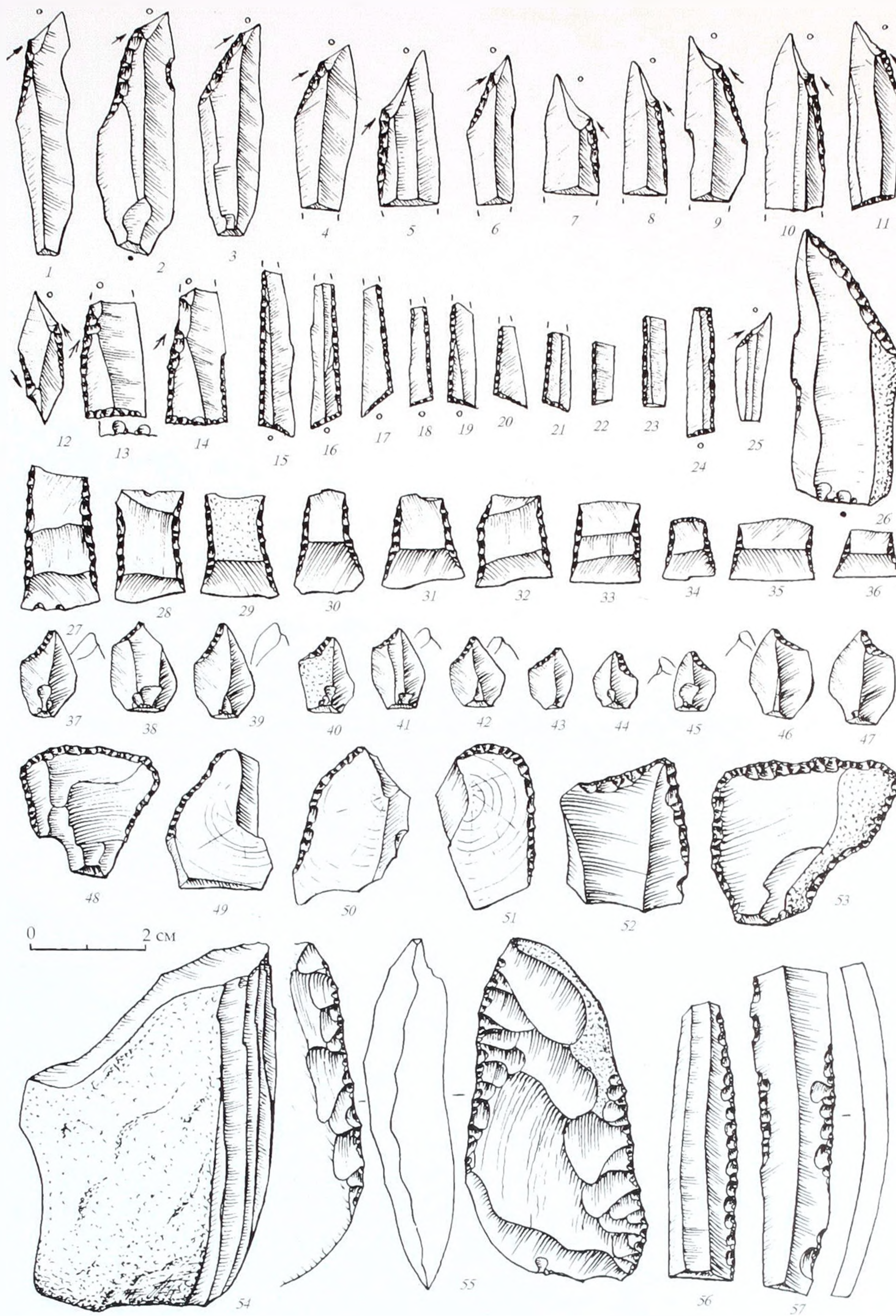
Рис. 30. Крем'яні вироби з яніславицької стоянки Сенчиці 5а на Верхній Прип'яті
