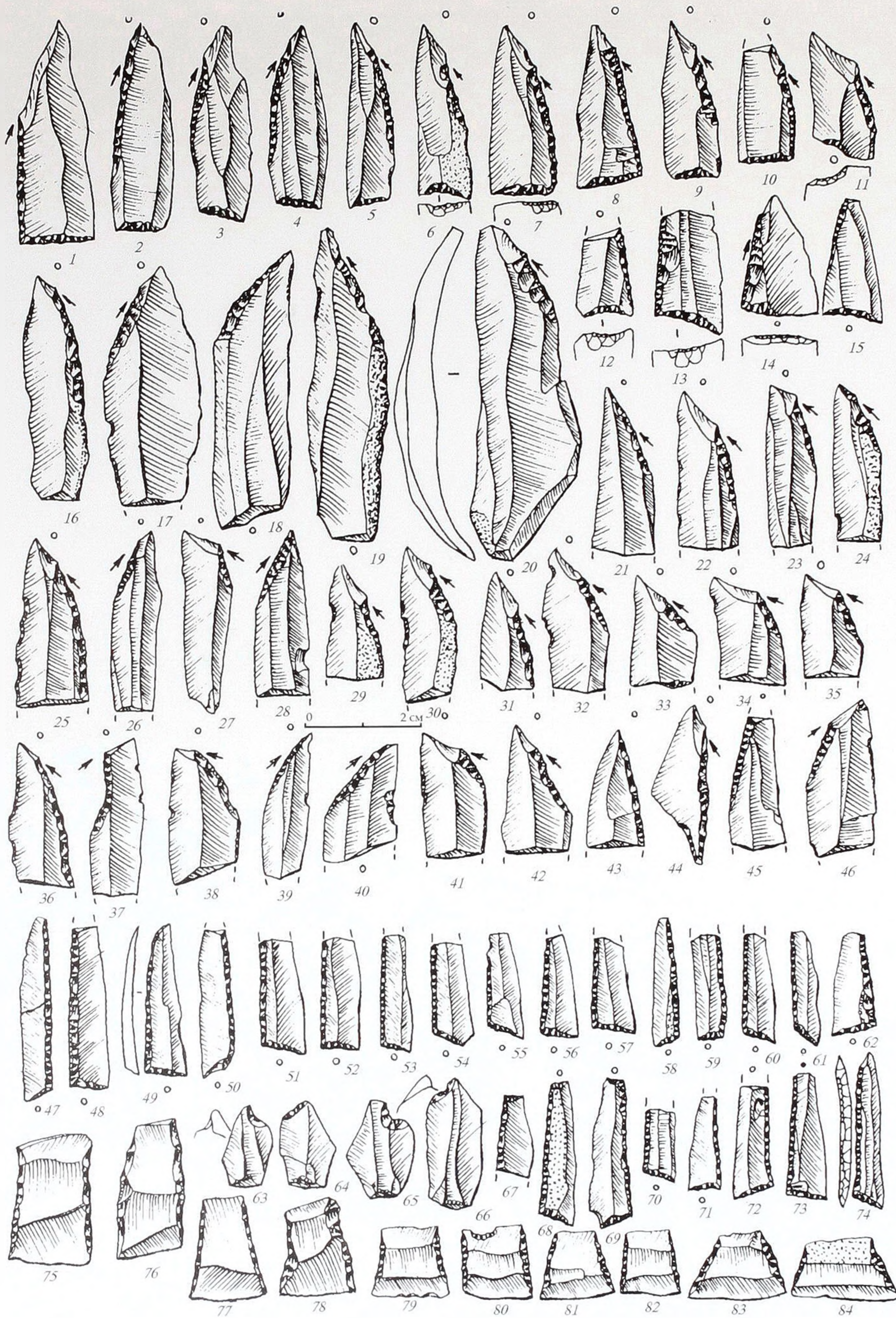
Рис. 31. Рудня 1. Мікроліти яніславицької культури
