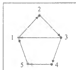
Рис. 2. Оргграф G
