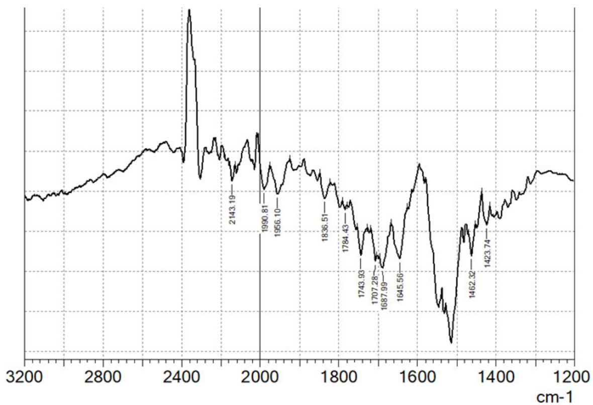
Рис. 1. FT-IR спектр пропускання для зразка №2.
