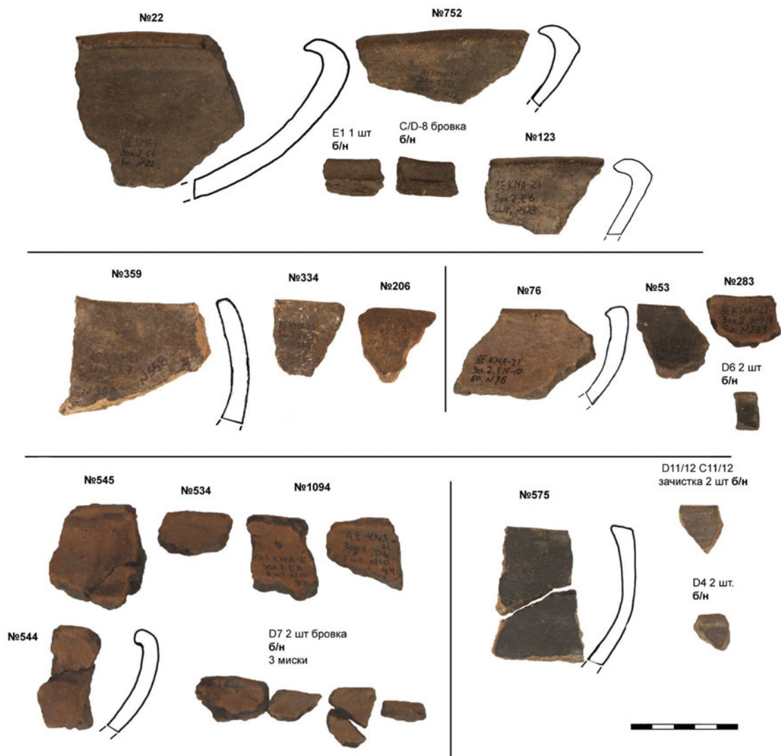
Рис. 41. Миски.
