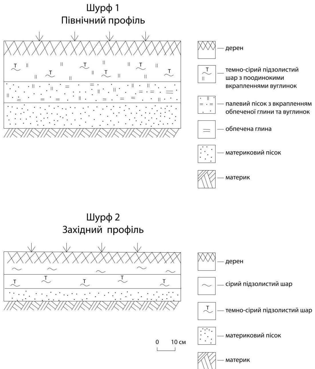
Рис. 74. Стратиграфія шурфів.
