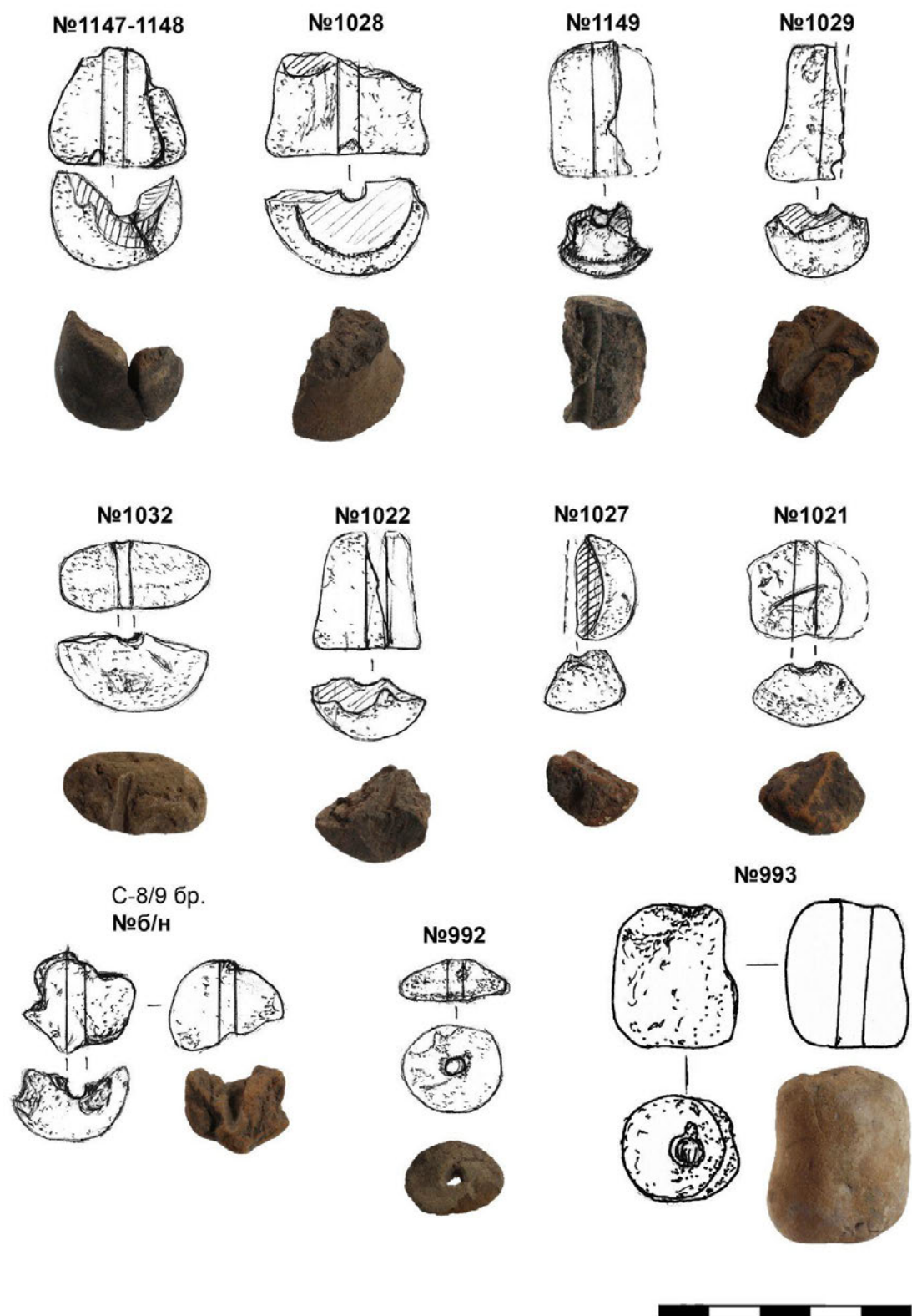
Рис. 62. Прясла IV.
