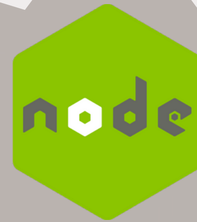
Node.js
