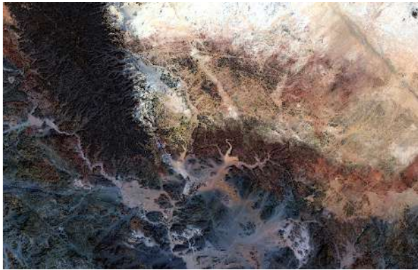
Комбінація B04, B03, B02
