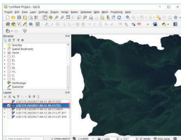
Природні кольори True Color Composite (TCC)
