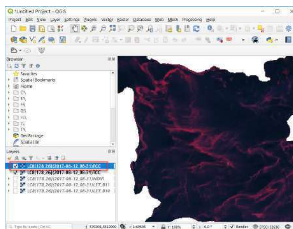
Штучні кольори False Color Composite (FCC)
