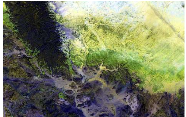
Комбінація B12, B11, B02
