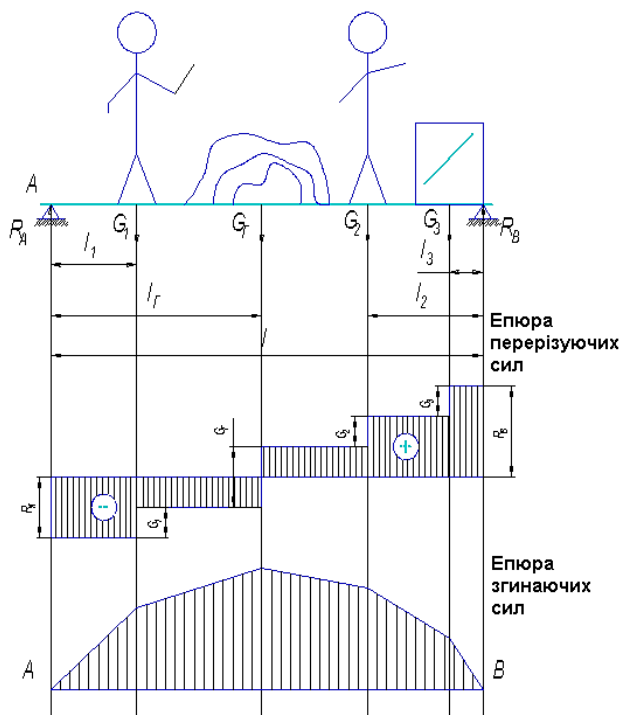
Рисунок 12.5 – Розрахунок навантаження настилу:
