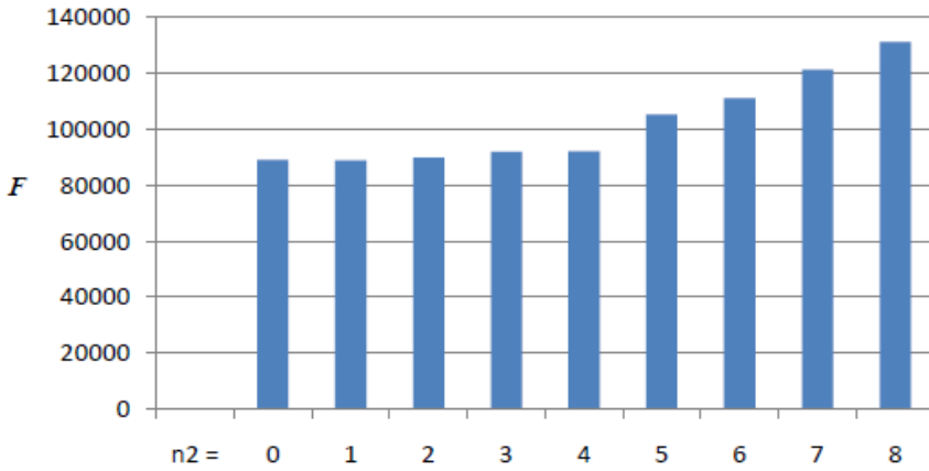
Рис. 6. Значення повних витрат у мережі при постійному значенні параметра w = 40 і зміні кількості вузлів другого типу, що включаються у мережу. Значення локальних мінімумів F до n_2 = 4 відстають дуже близько один від одного
