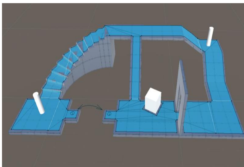
Рисунок 10 Unity Navigation System
