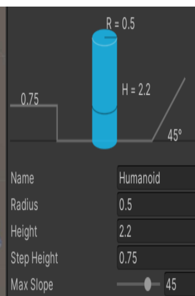
Рисунок 11 Agent Settings
