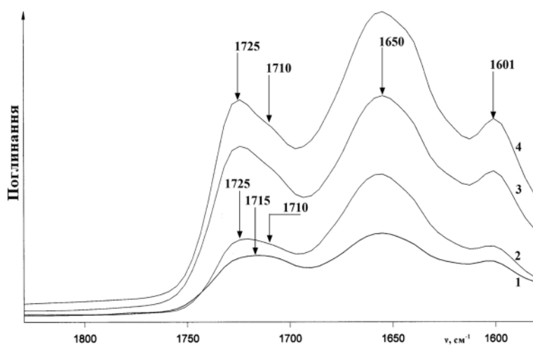
Рис. 6. Фрагменти ІЧ-спектрів полімерного матеріалу з амізоном після перебування в буферному розчині хімотрипсину: 1 – контроль, 2 – 2 тижні, 3 – 1 місяць, 4 – 6 місяців
