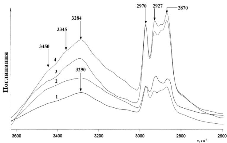
Рис. 5. Фрагменти ІЧ-спектрів полімерного матеріалу з амізоном після перебування в буферному розчині хімотрипсину: 1 – контроль, 2 – 2 тижні, 3 – 1 місяць, 4 – 6 місяців
