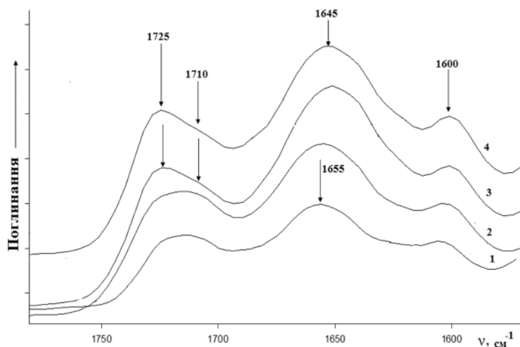
Рис. 4. Фрагменти ІЧ-спектрів полімерного матеріалу з амізоном після перебування в середовищі 199: 1 – контроль, 2 – 2 тижні, 3 – 1 місяць, 4 – 6 місяців
