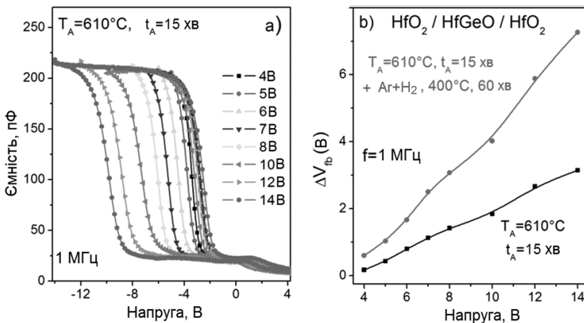
Рис. 7. Електричні властивості структури типу А, відпалених при T_A = 610^\circ C протягом 15 хв із подальшим додатковим відпалом у суміші азоту та водню при температурі 400^\circ C протягом 60 хв: а – C-V характеристики, одержані при різних напругах розгортки, виміряні на частоті 1 МГц; б – еволюція \Delta V_{fb}(V_G) при різних типах термічних обробок
