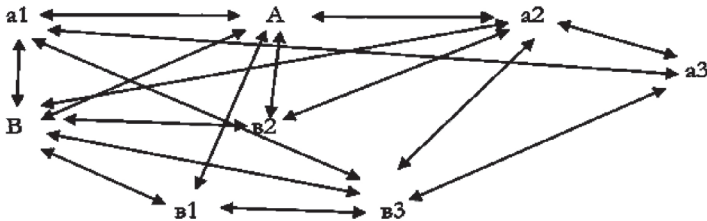
Рис. 4.1. Мережа-кліка
