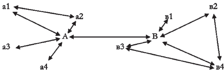
Рис. 4.2. Поліцефальна мережа
