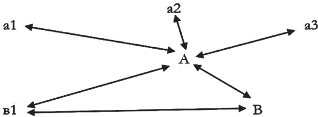
Рис. 4.3. Мережа-зірка
